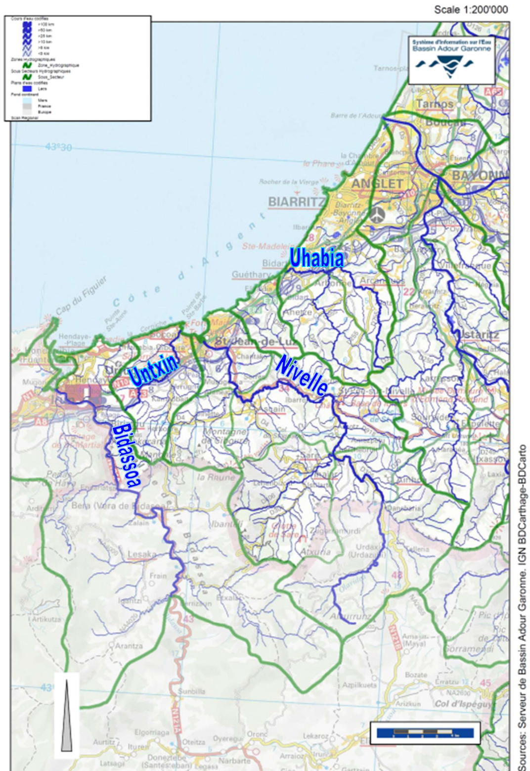
Figure 5 : Réseau hydrographique du Pôle territorial Sud Pays Basque (source SIE Adour Garonne)
